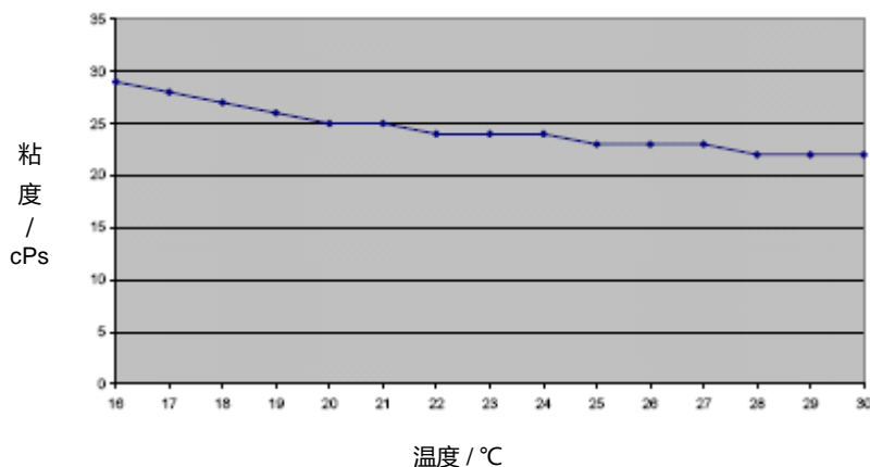
粘度 - 温度曲线 — CPL
